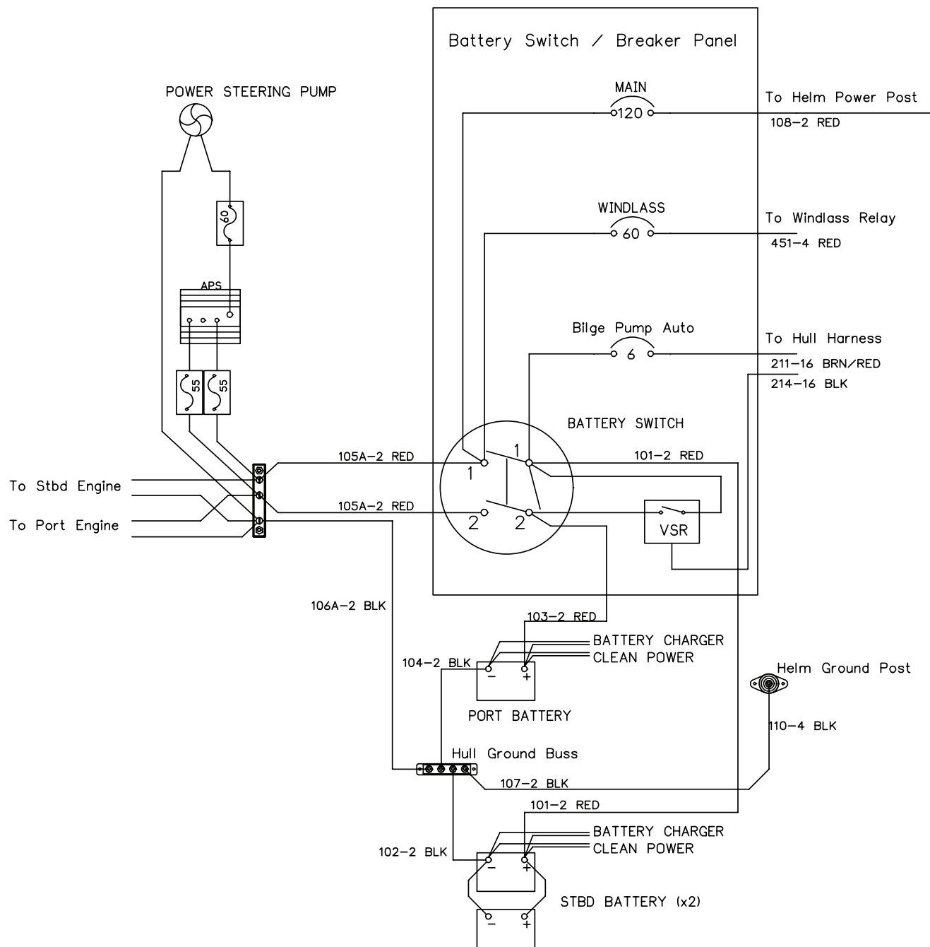
12 VDC Wiring Schematic Fig. 4.8.1
